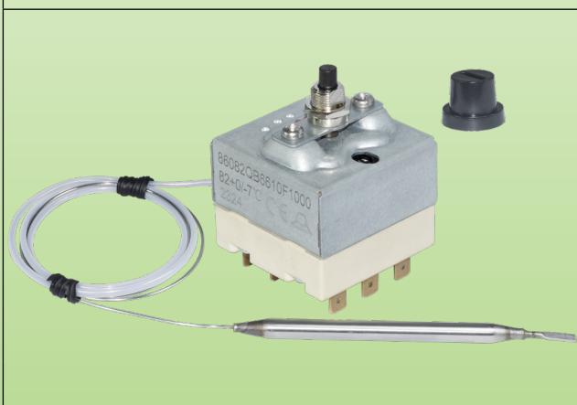
1: Etalonnage scellé; 2: Gainage du capillaire; 3: Bouton de réarmement manuel; 4: Capuchon du bouton de réarmement
